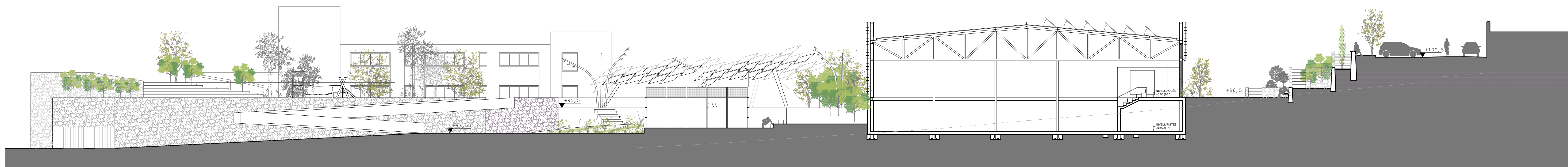
Sección B-B'
