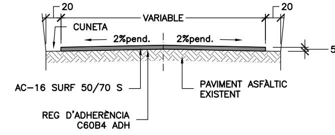
REFORÇ TIPUS 1 ESC. 1/50
